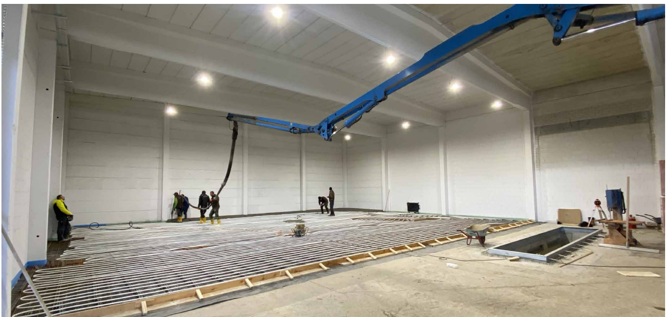
Hallenboden mit Fußbodenheizung
