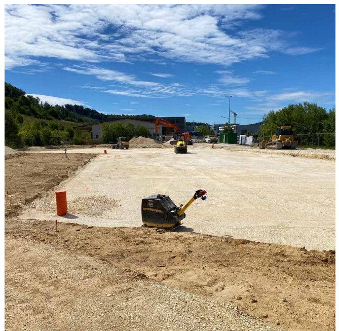
Erstellung Tragschicht
