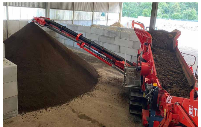
Aufbereitung Oberboden
